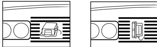
Antenă radar montată în poziție orizontală.
